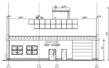
Projekt budynku OSP w Łośnie
