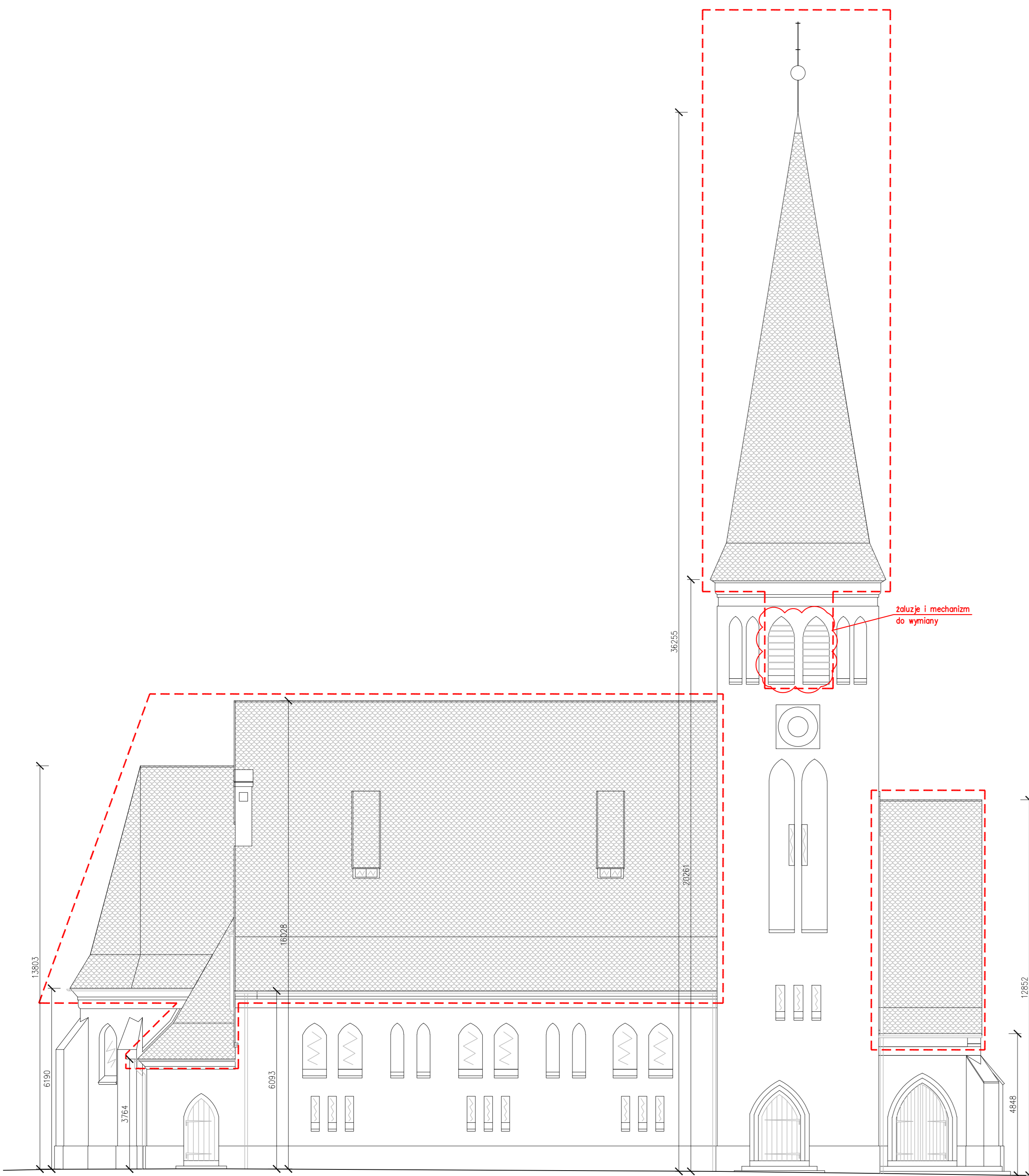
ELEVACJA POŁUDNIOWA
