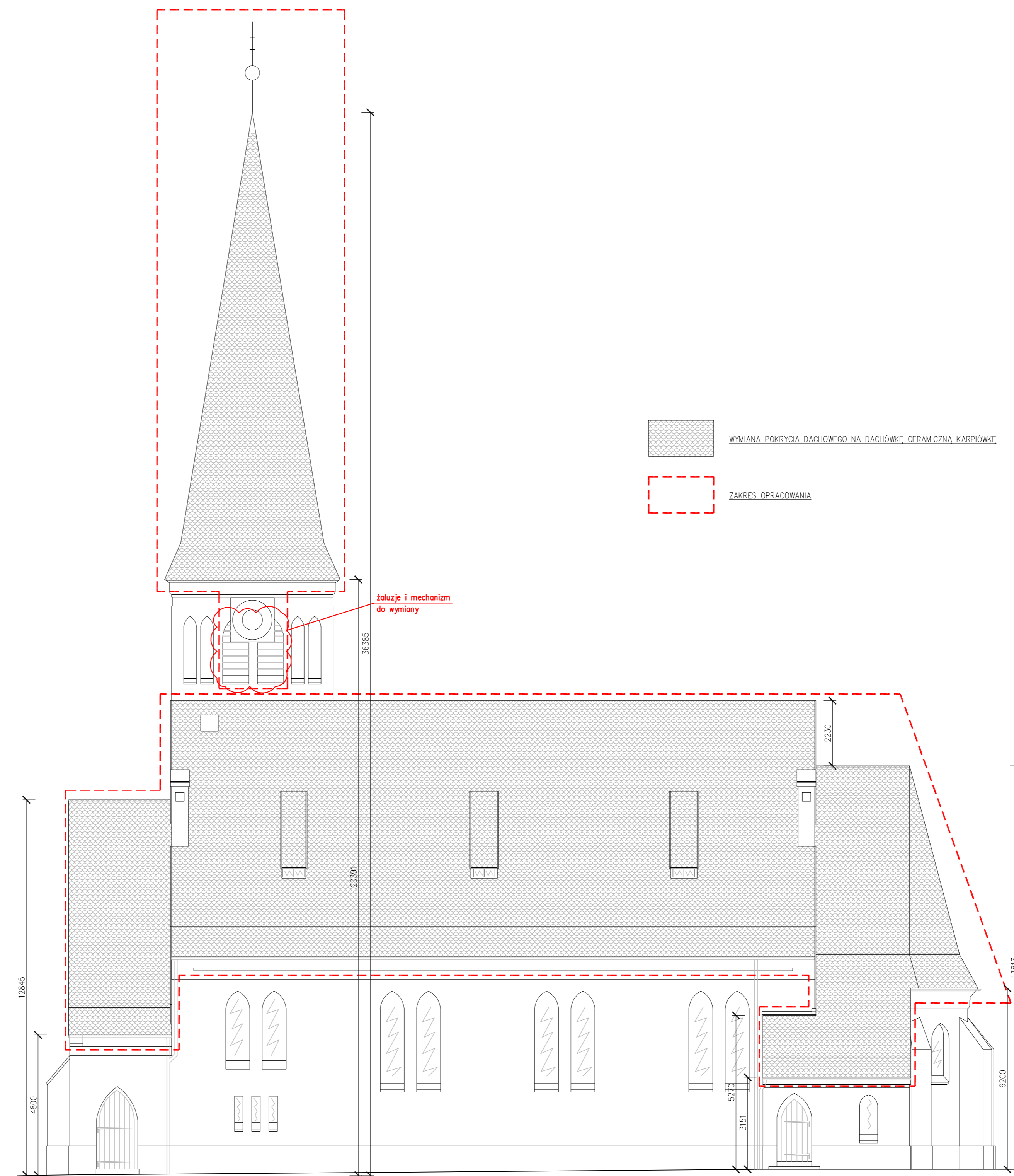
ELEVACJA PÓŁNOCNĄ
