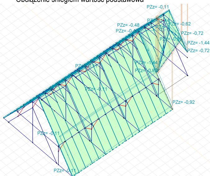
Obciążenie śniegiem zaspą śnieżną
