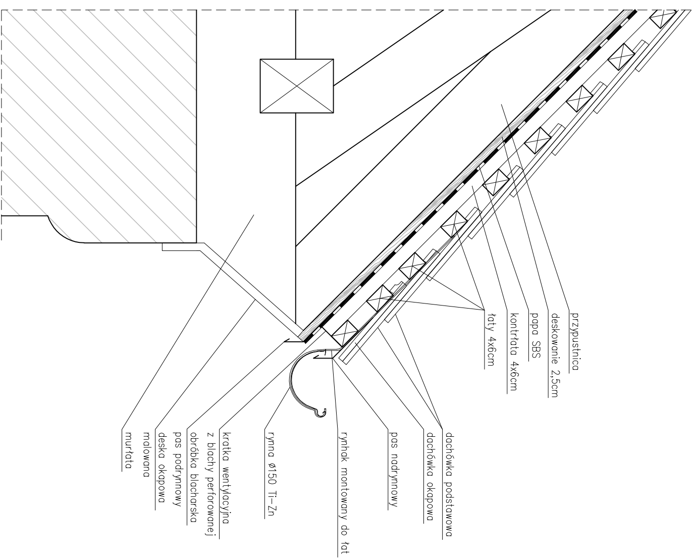
DETAL 1. Okap
