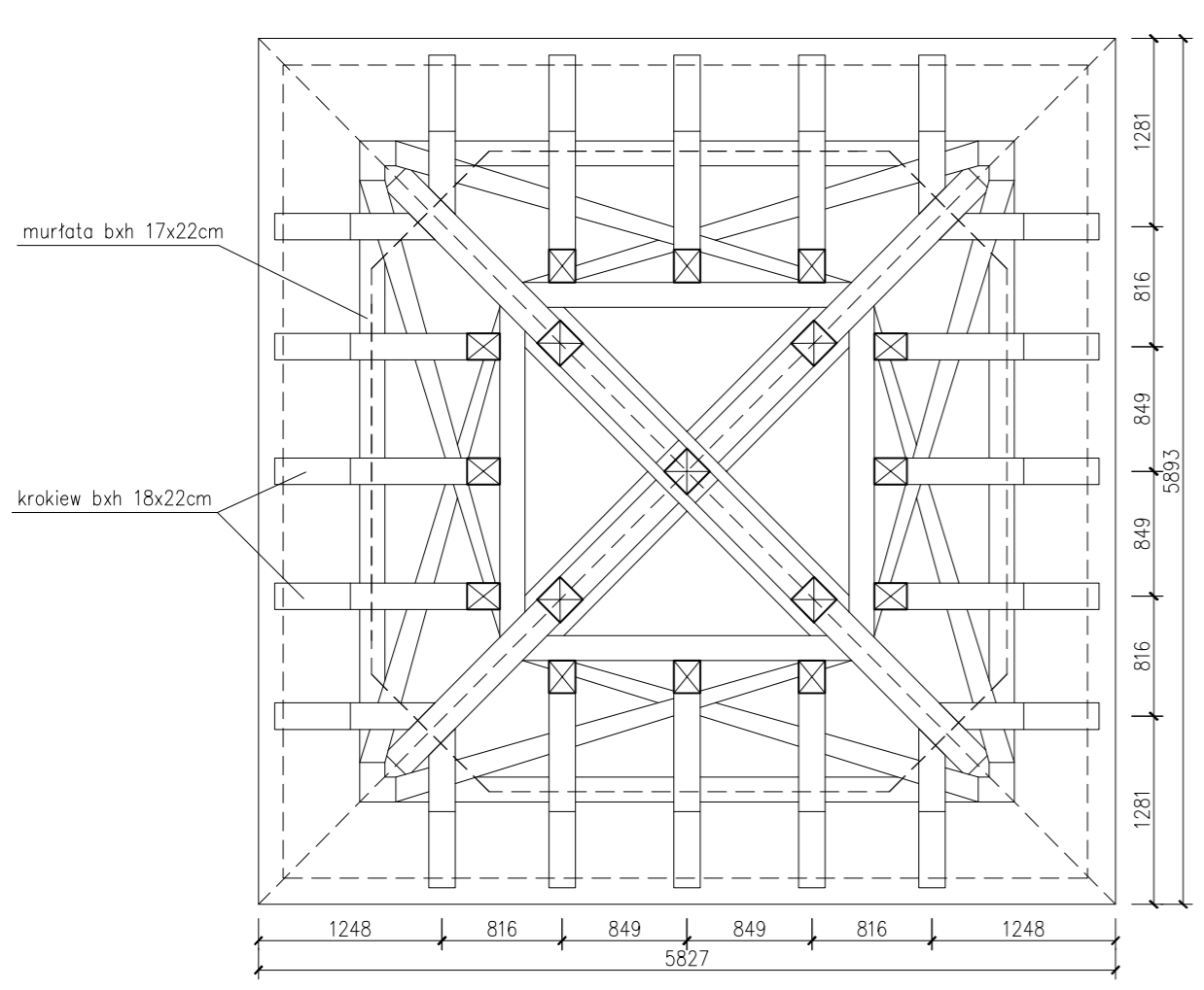
RZUT WIĘZBY DACHOWEJ WIEŻY
