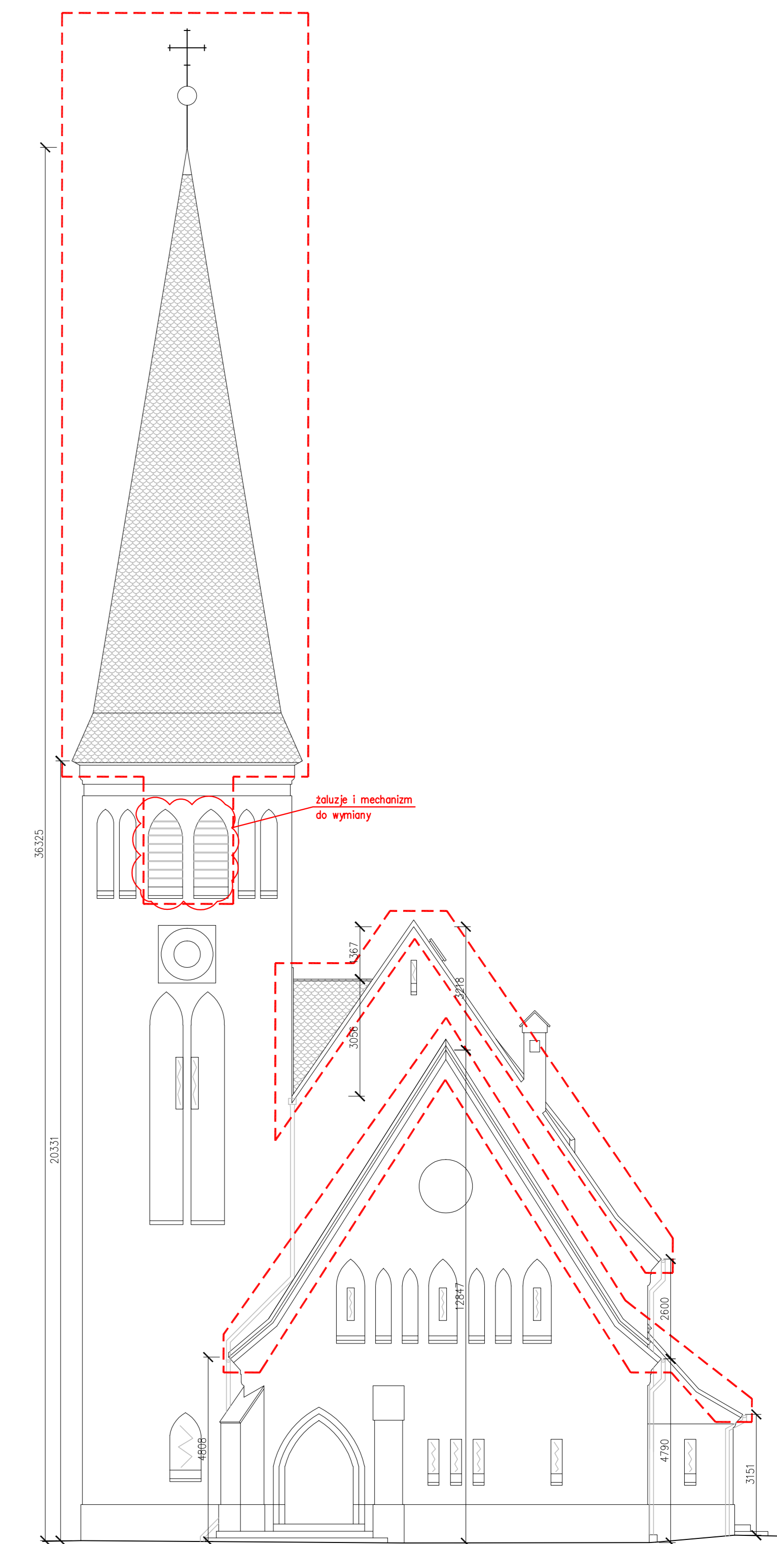
ELEVACJA ZACHODNIA
